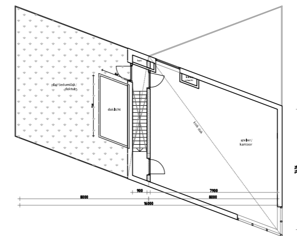
Dakopbouw 6500+P; atelier/werken
