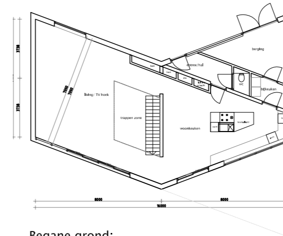
Begane grond; living, terras, keuken, entree en garage
